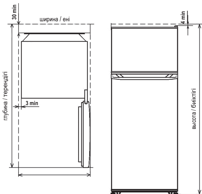
Рисунок Б.5 - Габаритное пространство - рабочие габаритные размеры Сурет Б.5 - Пішіндік кеңістік
