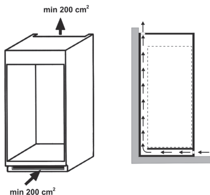
Рисунок Б.2 - Схема циркуляции воздуха вокруг холодильного прибора
