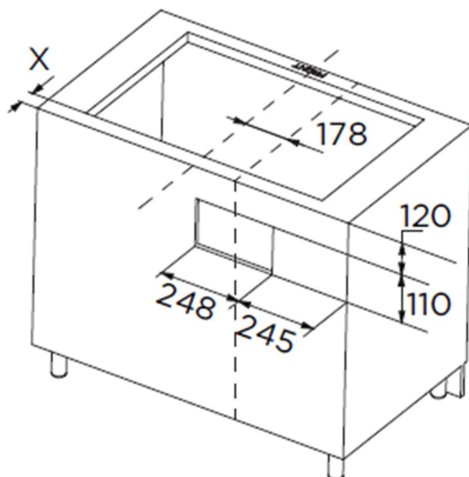
Вывод трубы без изгиба
